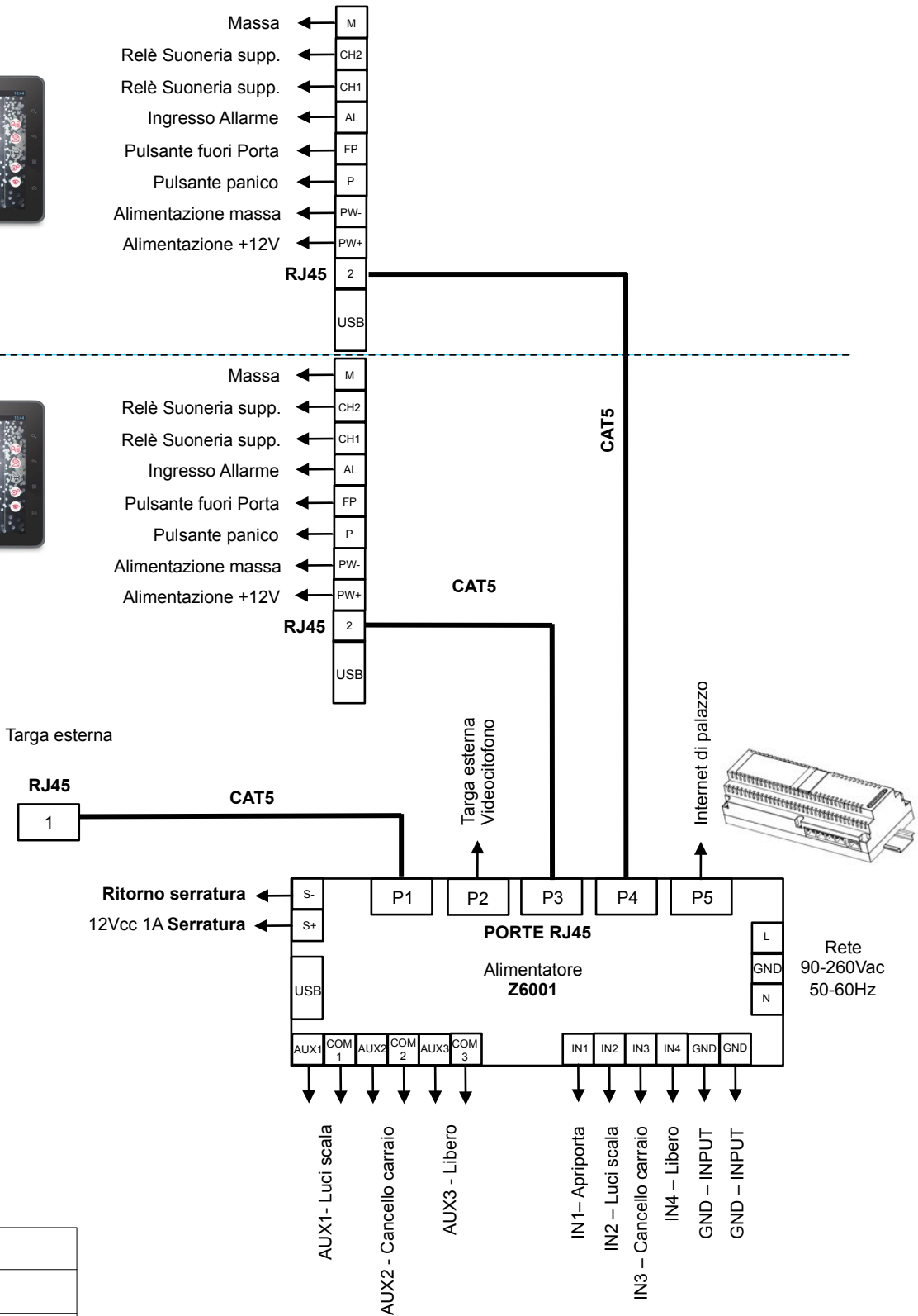
Videocitofono 2
