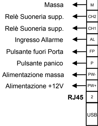
Videocitofono
